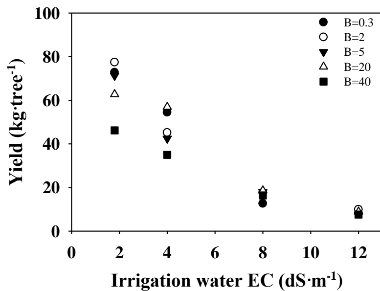
איור 4. יבול פירות תמרים מזן מלהול בשנת 2007, כתלות ברמת המליחות של תמיסת ההשקיה ( EC ) ברמות בורון ( B ) שונות
