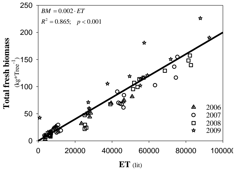
איור 3. משקל הביומסה הטרייה (יבול ועלווה) כתלות באוופוטנספירציה בכל שנה
